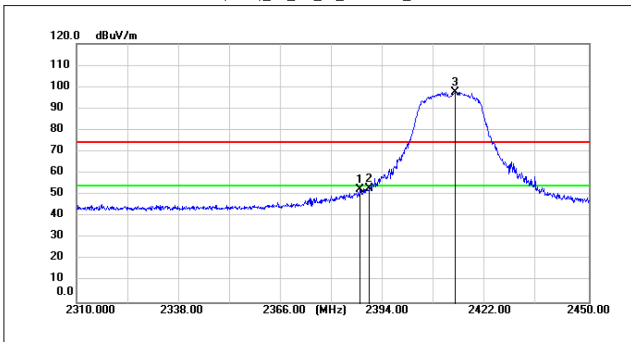
11n(HT20)_TX_CH_01_Horizontal_Peak
