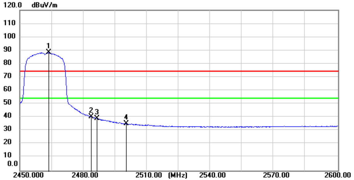
11n(HT20)_TX_CH_11_Horizontal_Average
