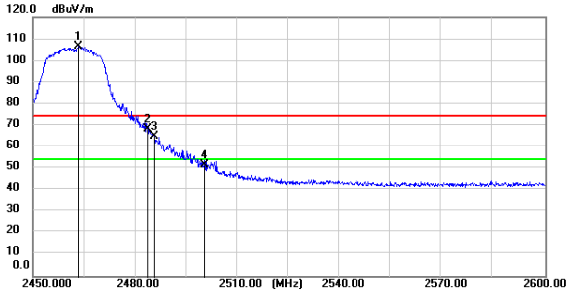
11n_HT(20M)_TX_CH_11_Horizontal
