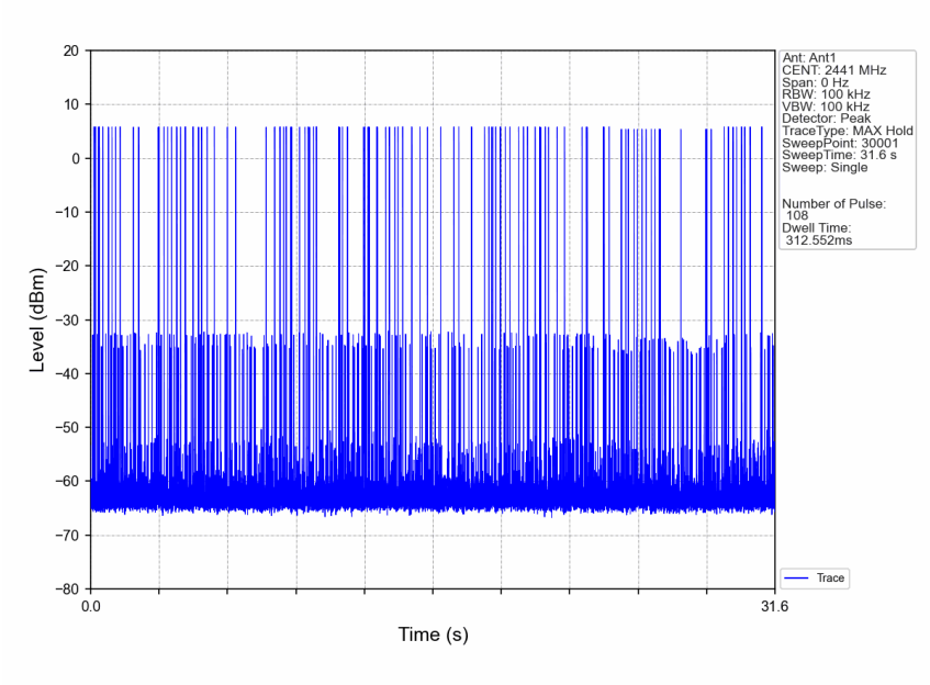
Pi/4DQPSK 2DH5 HOPP Ant1 NTNV
