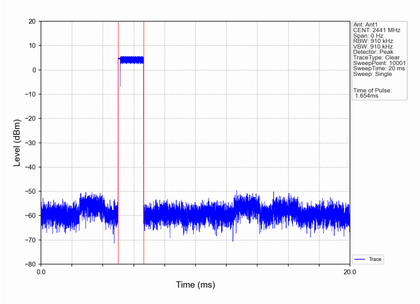
8DPSK 3DH3 HOPP Ant1 NTN
