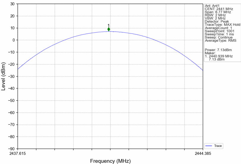
8DPSK 3DH5 MCH 2441MHz Ant1 NTNV
