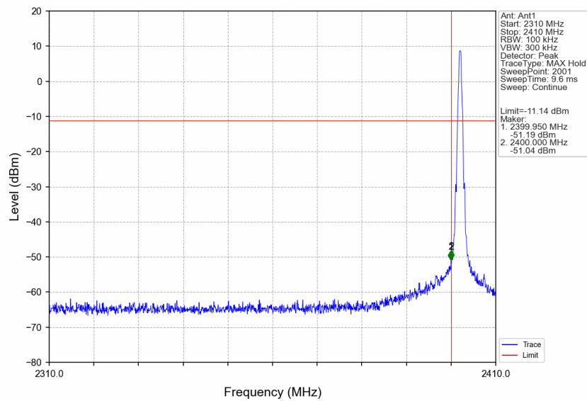
GFSK DH5 LCH 2402MHz Ant1 NTN
