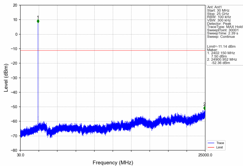
GFSK DH5 LCH 2402MHz Ant1 NTN
