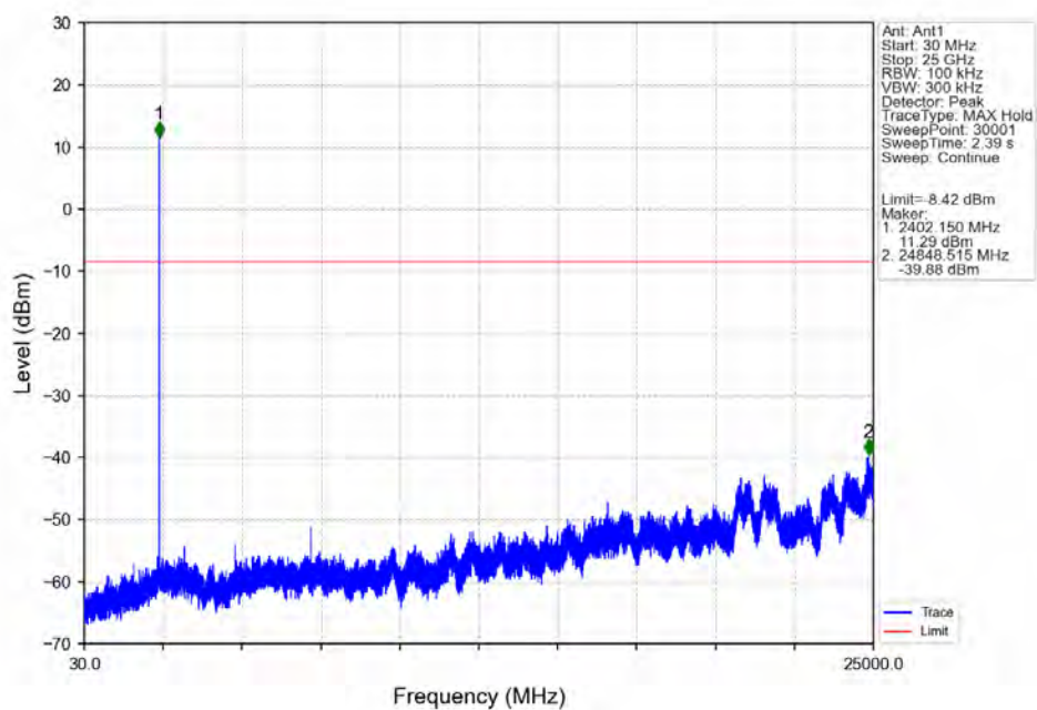
GFSK DH5 LCH 2402MHz Ant1 NTN
