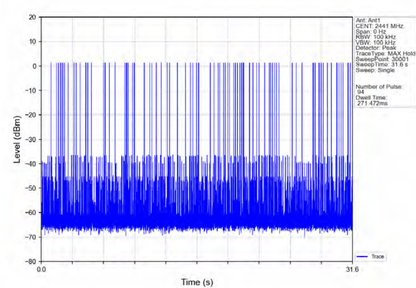
GFSK_DH5_HOPP_Ant1_NTNV
