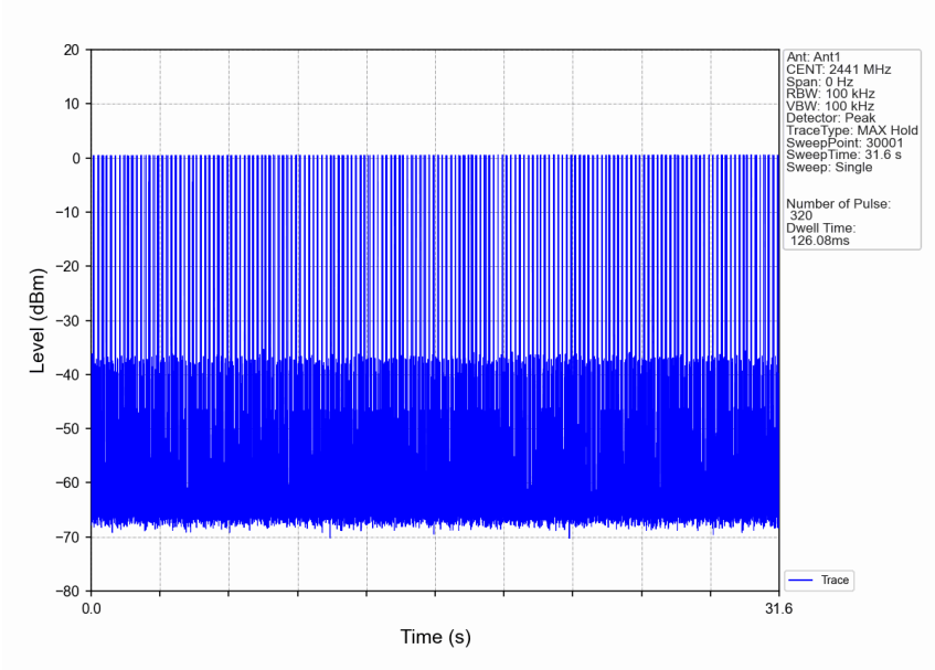
Pi/4DQPSK_2DH1_HOPP_Ant1_NTNV
