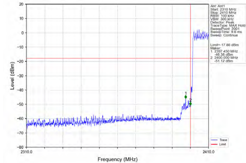
Pi/4DQPSK_2DH5_HOPP_Ant1_NTNV
