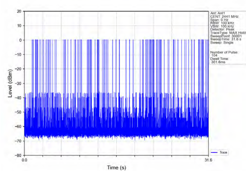
8DPSK_3DH5_HOPP_Ant1_NTNV
