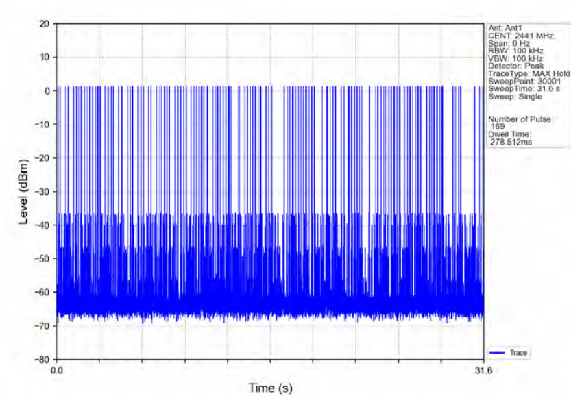
GFSK_DH3_HOPP_Ant1_NTNV
