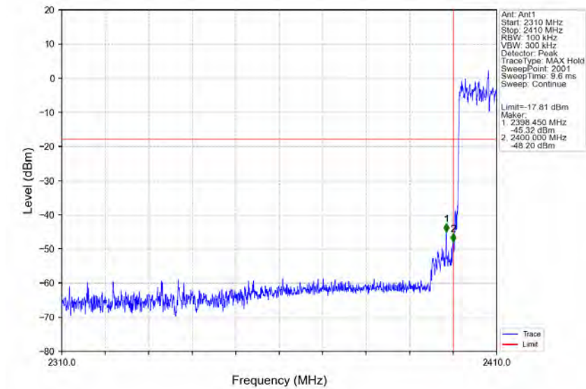
Pi/4DQPSK_2DH5_HOPP_Ant1_NTNV
