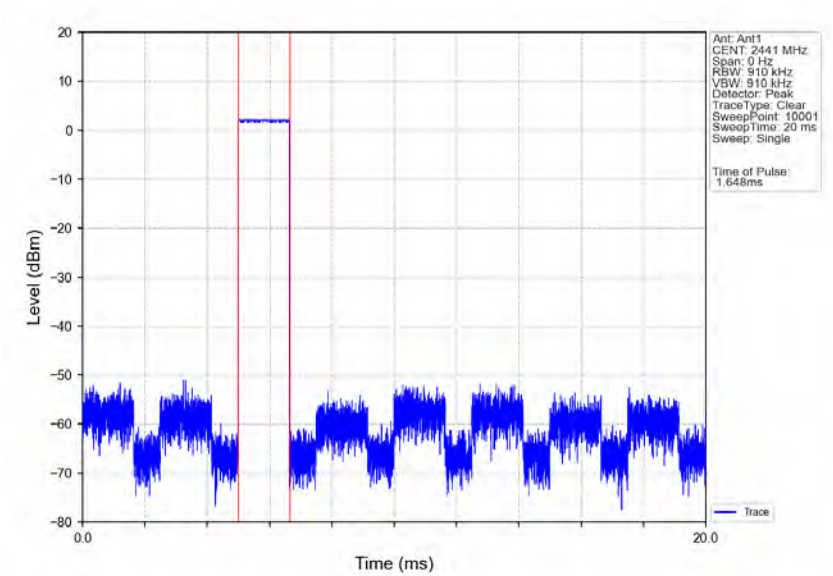
GFSK_DH3_HOPP_Ant1_NTNV
