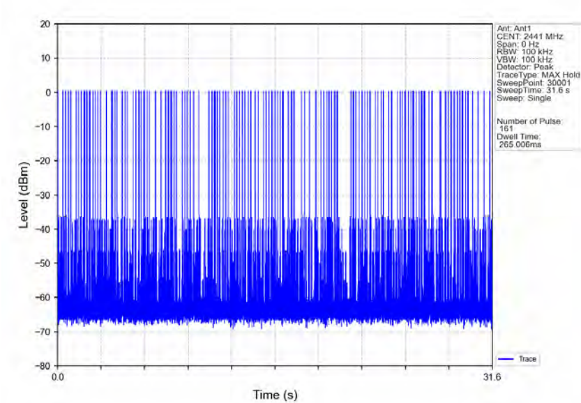
8DPSK_3DH3_HOPP_Ant1_NTNV
