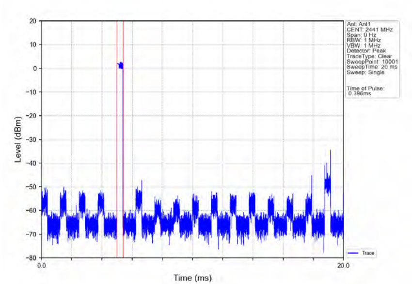
8DPSK_3DH1_HOPP_Ant1_NTNV
