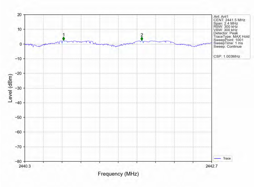
8DPSK_3DH5_HOPP_Ant1_NTNV
