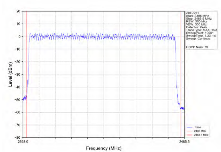
8DPSK_3DH5_HOPP_Ant1_NTNV
