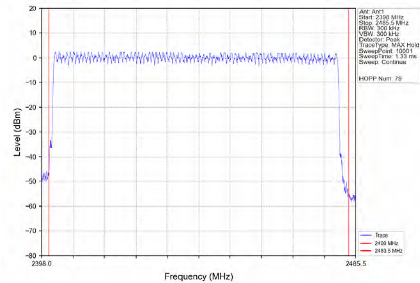
8DPSK_3DH5_HOPP_Ant1_NTNV
