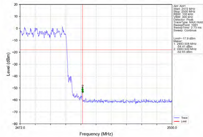
8DPSK_3DH5_HOPP_Ant1_NTNV
