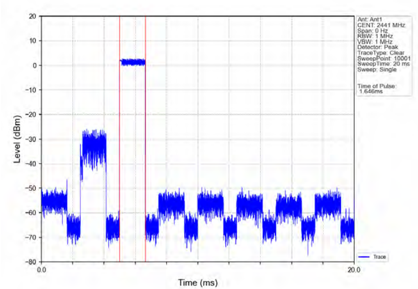
8DPSK_3DH3_HOPP_Ant1_NTNV
