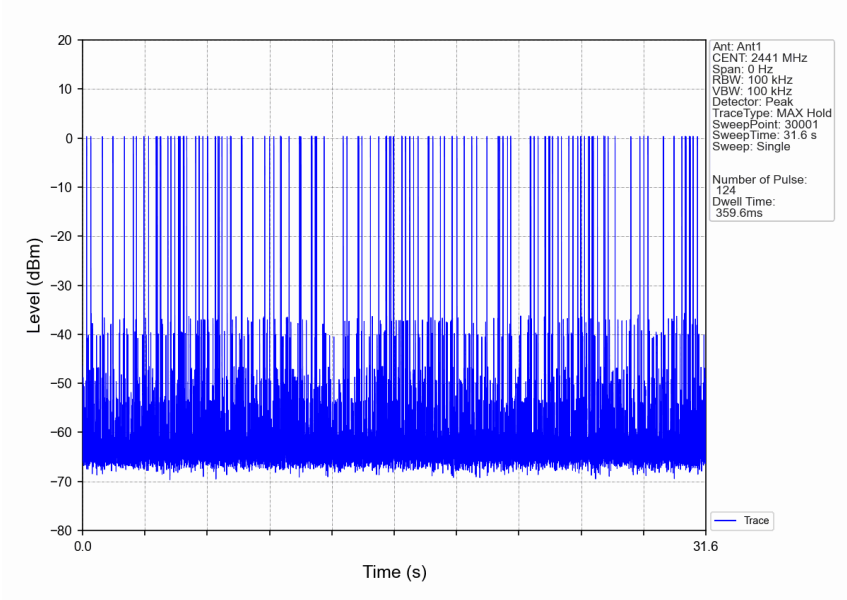
Pi/4DQPSK_2DH5_HOPP_Ant1_NTNV
