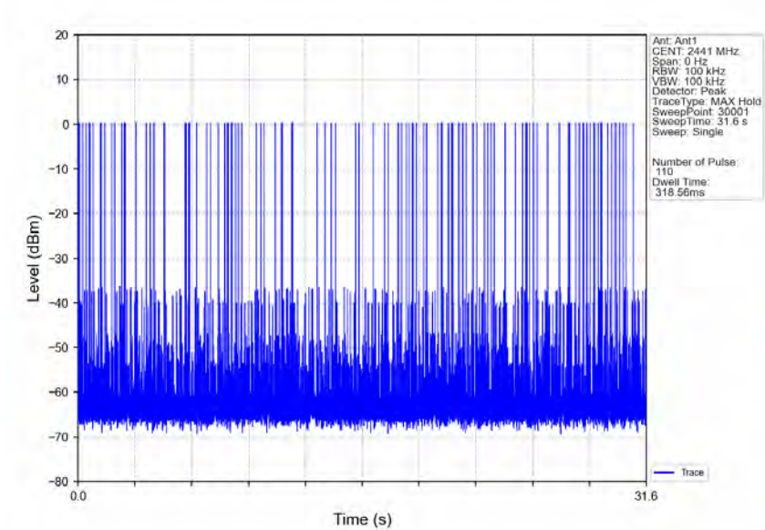
Pi/4DQPSK_2DH5_HOPP_Ant1_NTNV
