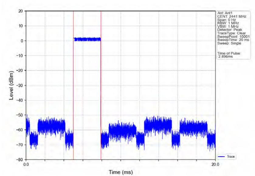
Pi/4DQPSK_2DH5_HOPP_Ant1_NTNV
