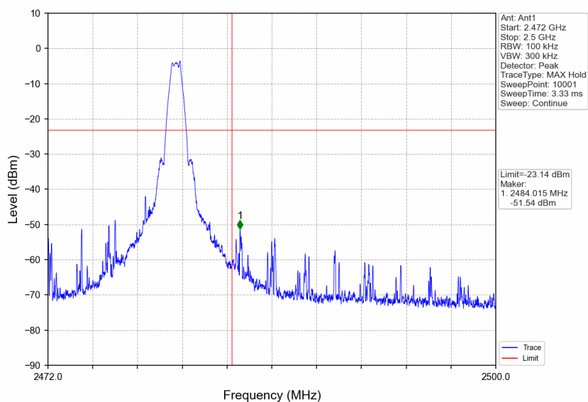
1M_HCH_2480MHz_DataRate=_Ant1_NTNV
