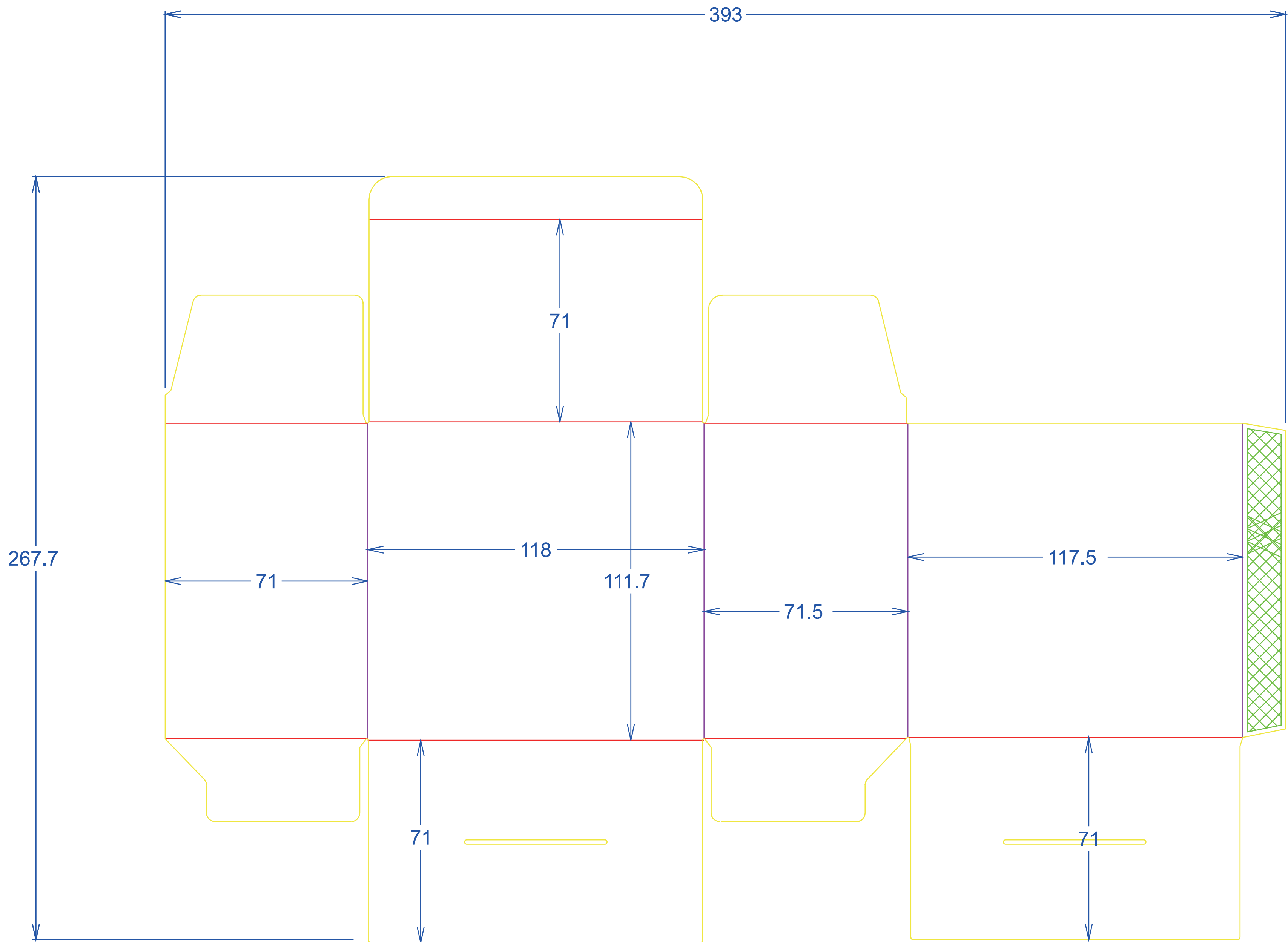
部件名称: 封套 材质: 350g光刻纸
