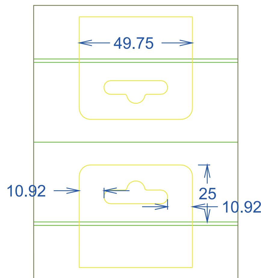
部件名称: 挂钩 材质: 350g光刻纸对裱模切
