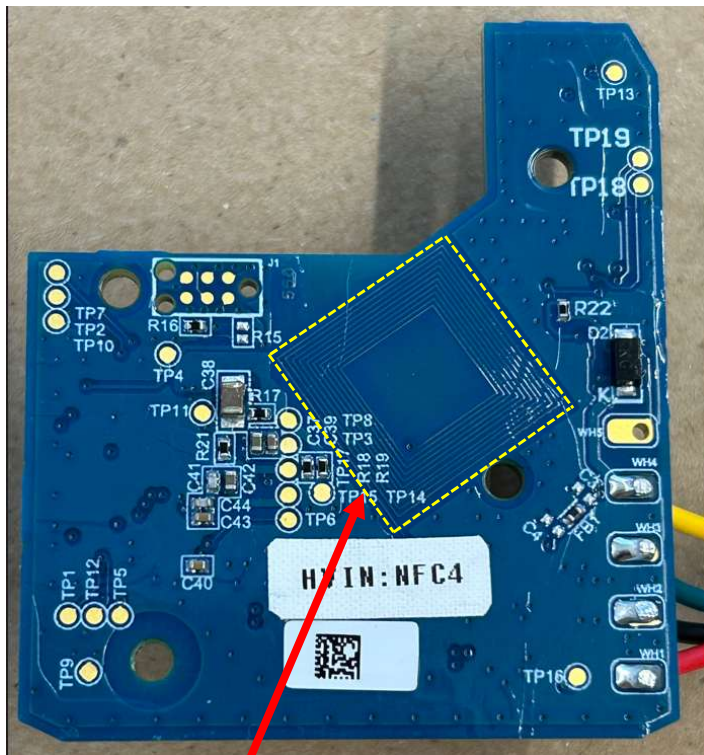
Antenna
