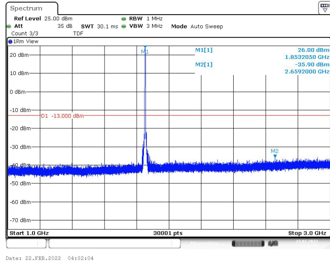
Band2-9262-4-1000~3000MHz
