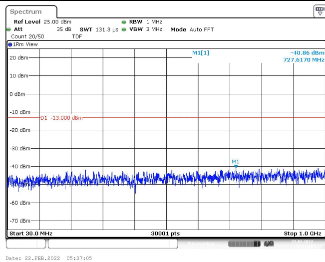
Band2-9538-1-30~1000MHz
