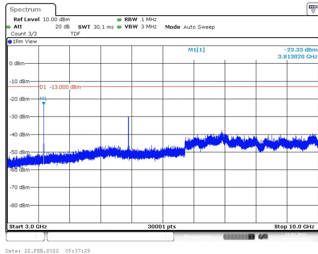
Band2-9538-1-3000~10000MHz
