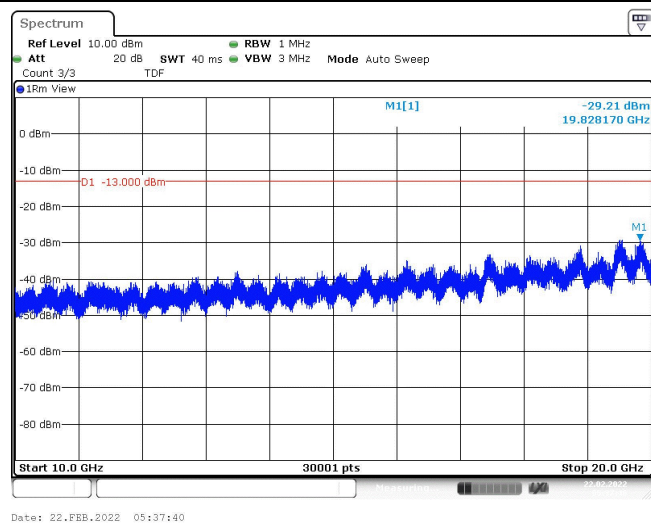
Band2-9538-1-10000~20000MHz
