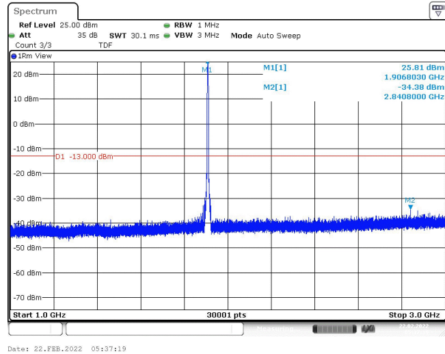
Band2-9538-1-1000~3000MHz
