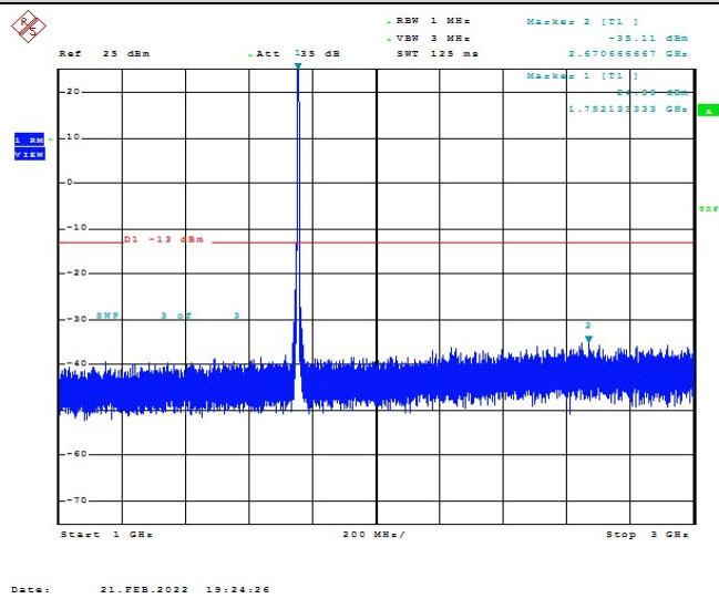
Band4-1513-3-1000~3000MHz
