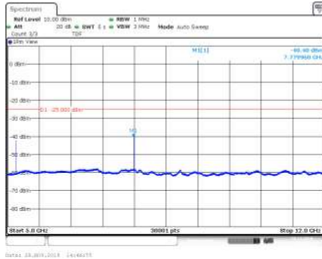
Band41_15MHz_QPSK_40690_1RB#0
