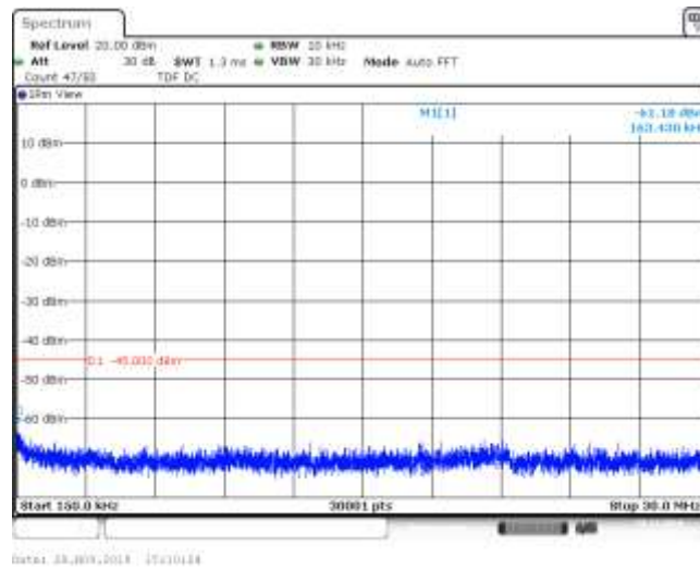
Band41_20MHz_QPSK_40690_1RB#0
