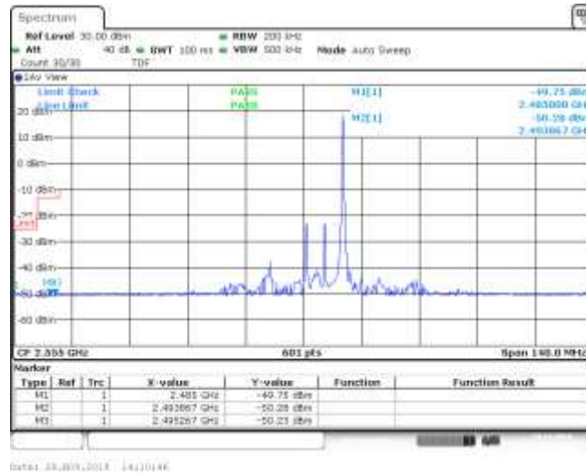
Band41_10MHz_QPSK_40290_50RB#0
