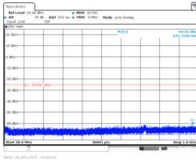
Band41_10MHz_QPSK_41190_1RB#0
