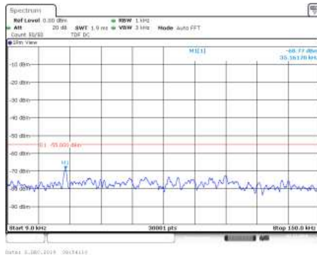
Band41_10MHz_QPSK_40690_1RB#0
