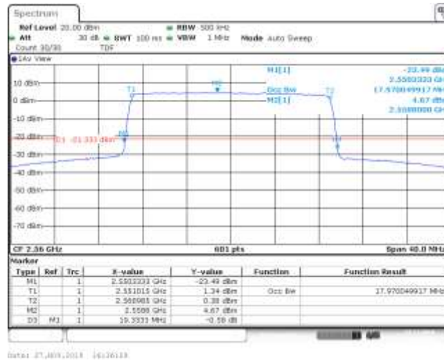
Band7_20MHz_16QAM_21350_100RB#0
