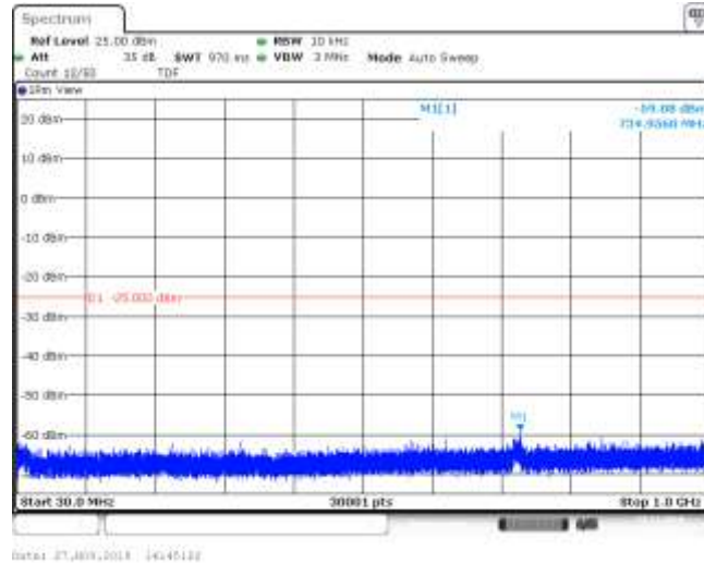
Band7_20MHz_16QAM_20850_1RB#0
