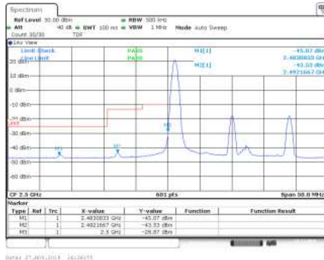
Band7_20MHz_QPSK_20850_1RB#49
