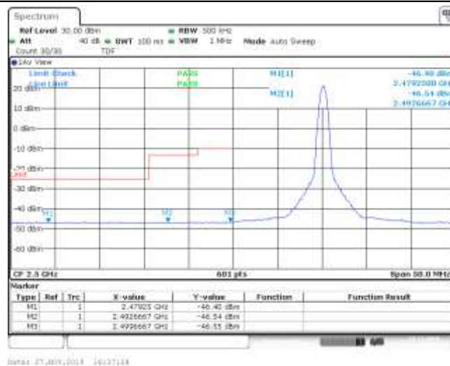
Band7_20MHz_QPSK_20850_1RB#49
