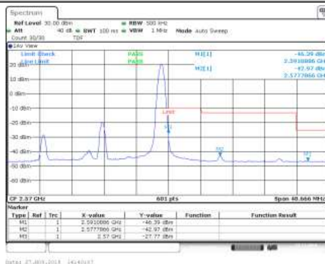
Band7_20MHz_QPSK_21350_1RB#99
