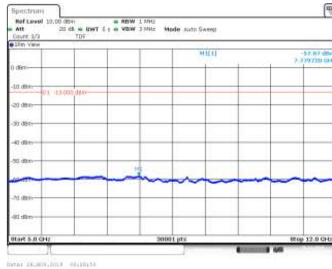
Band5_3MHz_16QAM_20635_1RB#0
