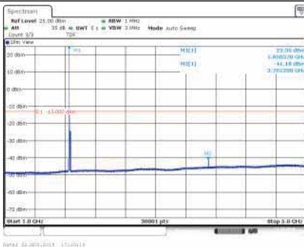
Band2_10MHz_QPSK_18650_1RB#0
