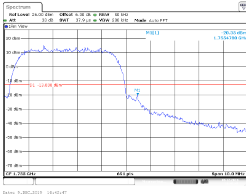
Band IV-1513-HSUPA_Sub3
