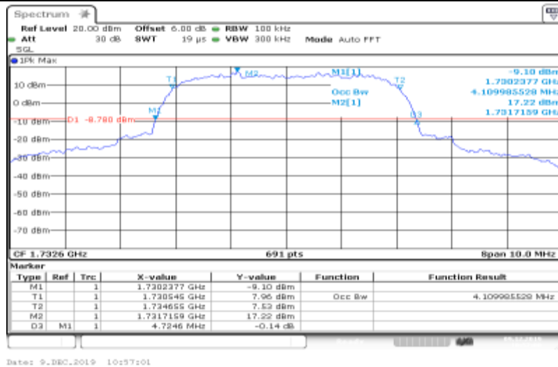
Band IV-1413-HSUPA_Sub2
