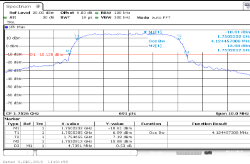
Band IV-1513-HSUPA_Sub3
