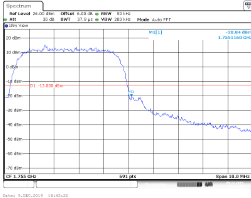
Band IV-1513-HSUPA_Sub2
