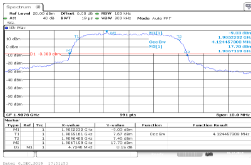
Band II-9538-HSUPA_Sub2
