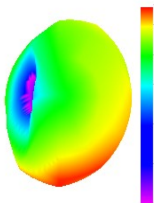
2500.000MHz E1
