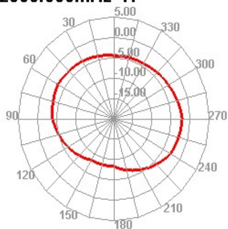
2500.000MHz H
