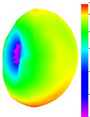
2400.000MHz E1
