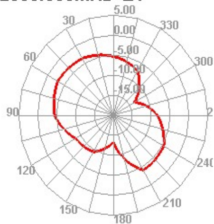
2500.000MHz E1
