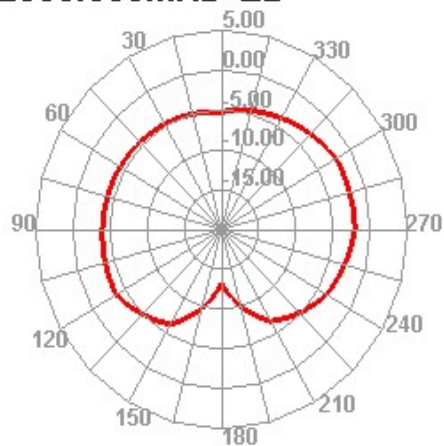
2500.000MHz E2
