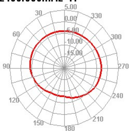
2400.000MHz E2
