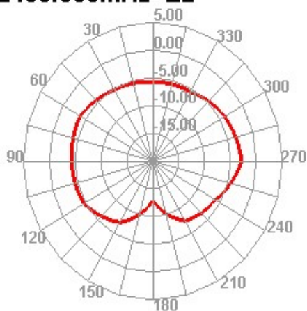
2450.000MHz H
