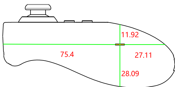
发送端边缘到外壳表面距离 示意简图 单位: mm
