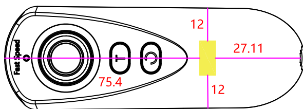
发送端边缘到外壳表面距离 示意简图 单位: mm
