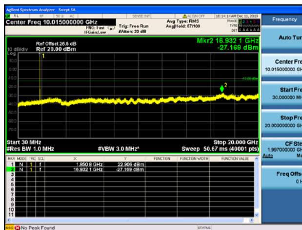
Band2 / 20MHz / Low CH / 64QAM
