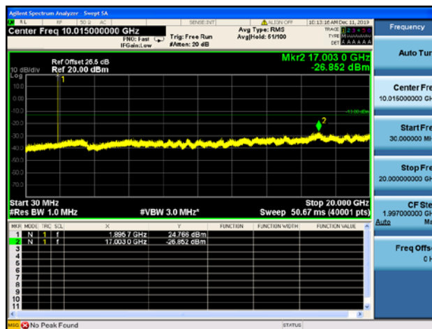
Band2 / 20MHz / Low CH / QPSK
