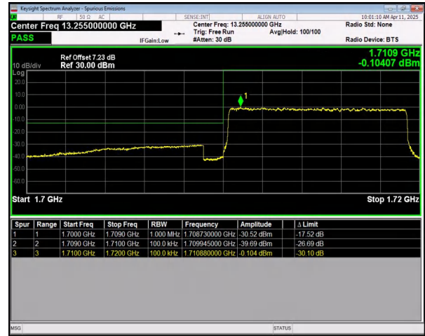
n66 SCS=15kHz DFT_256QAM BW=10MHz LowChannel=343000 RB=50@0
