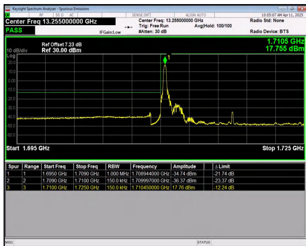
n66 SCS=15kHz DFT_256QAM BW=15MHz LowChannel=343500 RB=1@0
