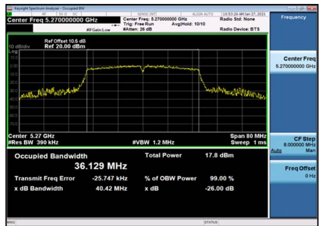
U-NII-2a 26dB Bandwidth-802.11ac(40MHz),5270MHz,Ant1
