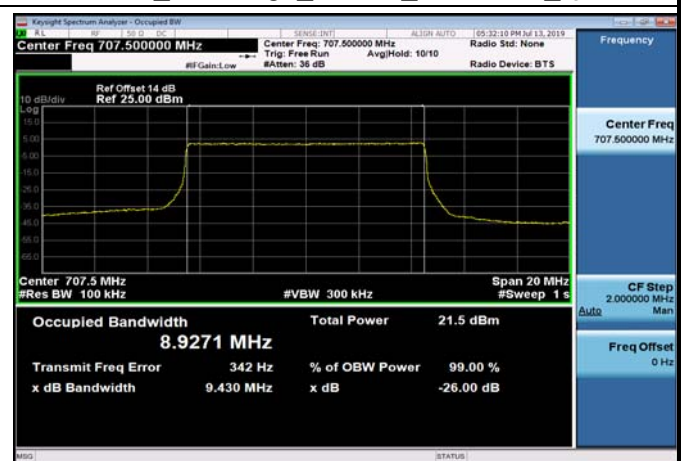
FDD12_MidRange_10MHz_707.5MHz_Q16
