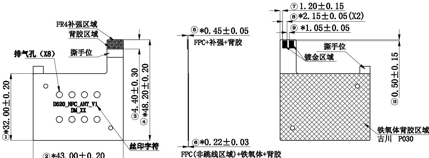
正面 (A面)
