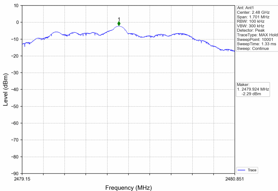
2M_HCH_2480MHz_DataRate=_Ant1_NTNV
