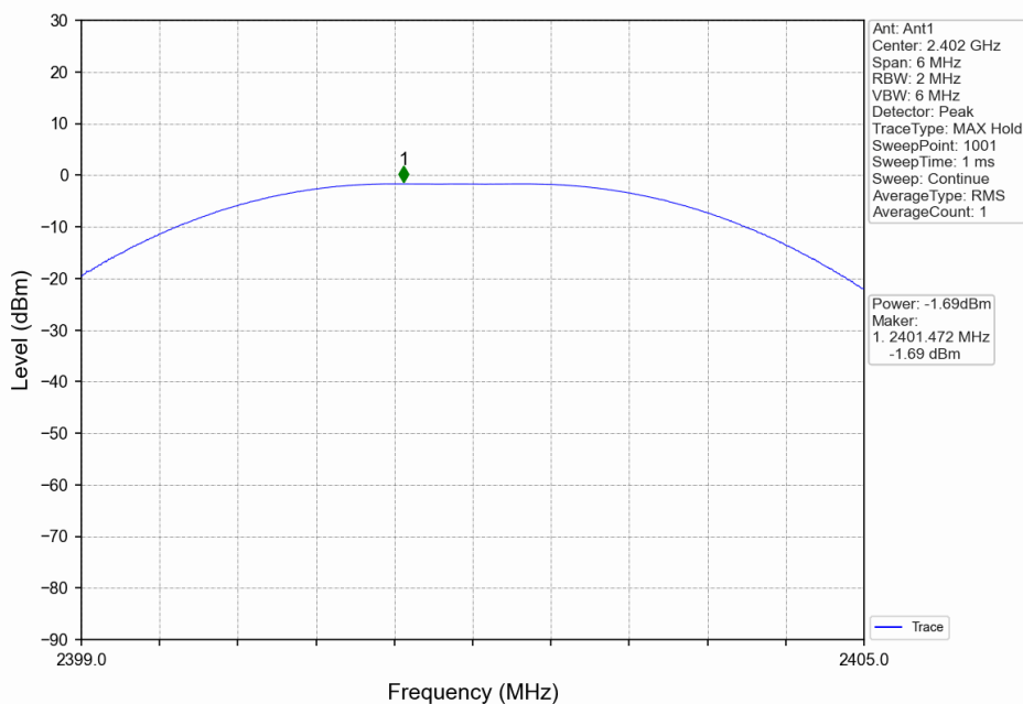
2M_LCH_2402MHz_DataRate=_Ant1_NTNV
