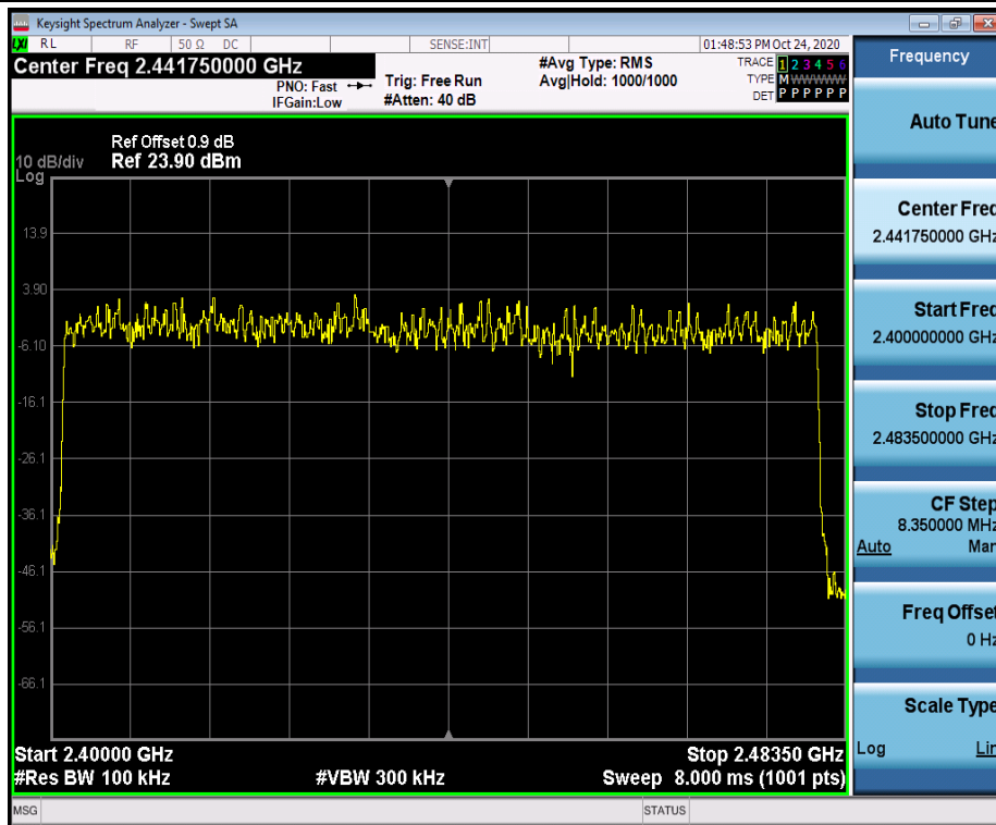
3DH5_Ant1_Hop
