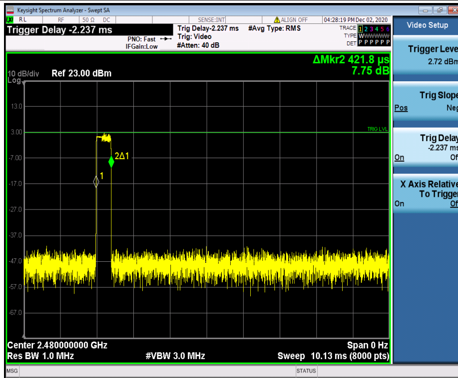
3DH1_Ant1_Hop_2480
