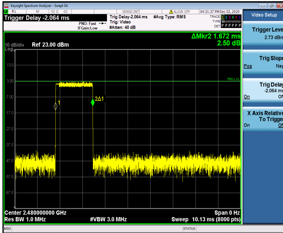
3DH3_Ant1_Hop_2480
