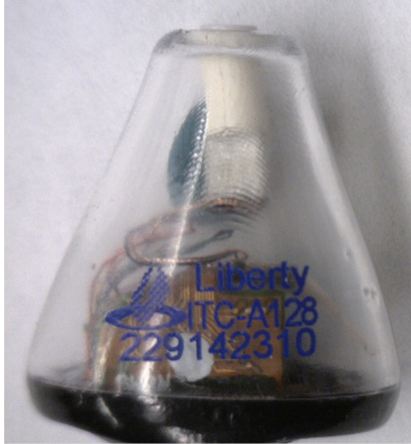
ITC-A (Android)
