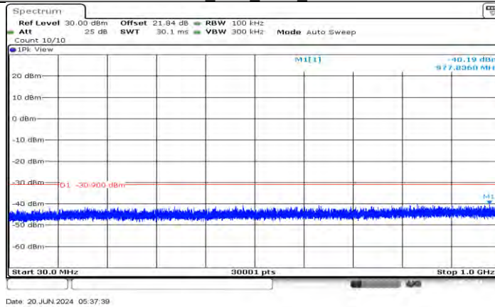
11AX40SISO_Ant1_2452_30~1000
