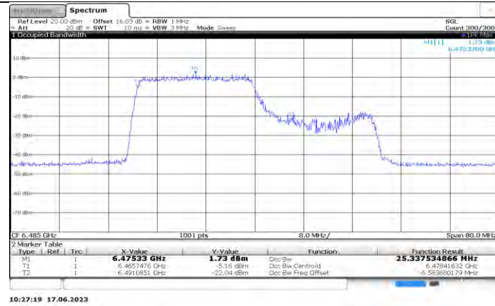
11AX40MIMO_Ant0_6485_242Tone_RU61
