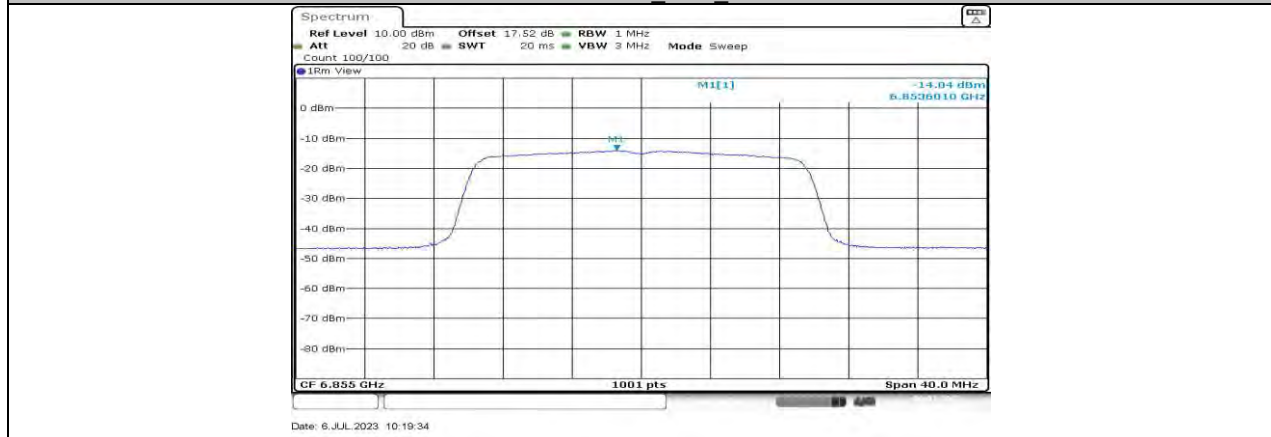
11AX20MIMO_Ant0_6855
