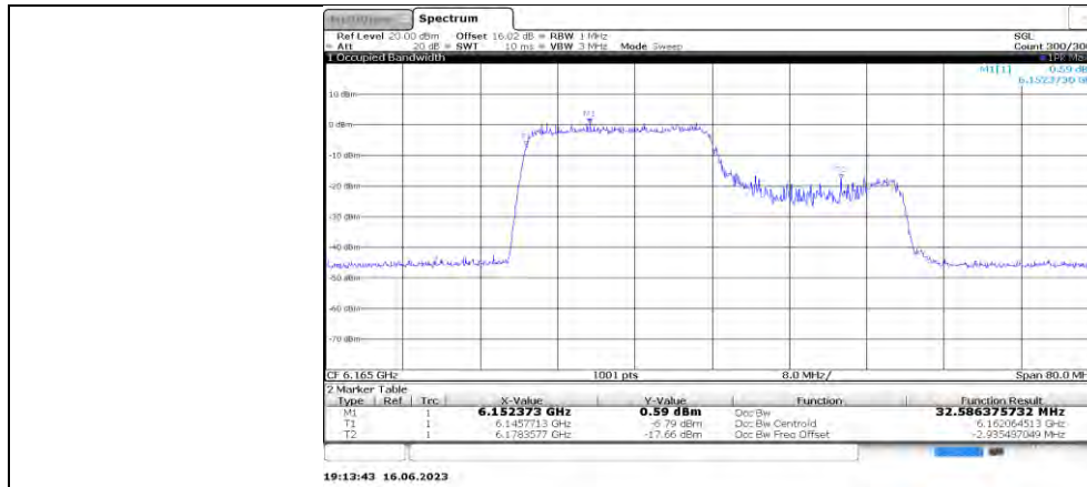
11AX40MIMO_Ant0_6165_242Tone_RU61
