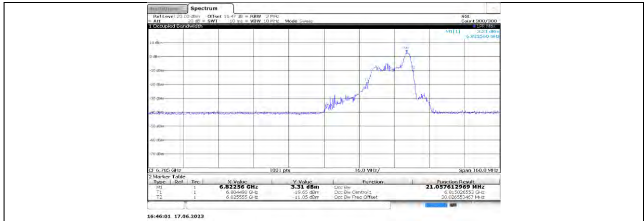
11AX80MIMO_Ant0_6785_26Tone_RU36
