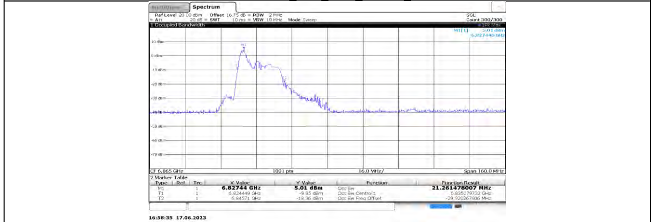
11AX80MIMO_Ant0_6865_26Tone_RU0
