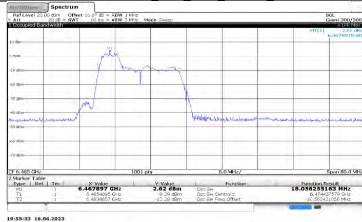
11AX40MIMO_Ant1_6485_52Tone_RU37
