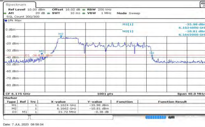
11AX20MIMO Ant1 6175 52Tone RU37
