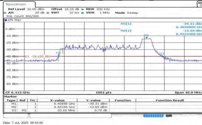
11AX20MIMO Ant0 6415 26Tone RU8
