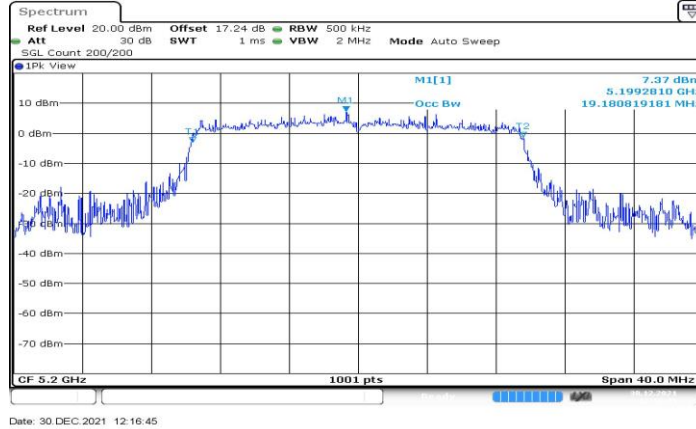
11AX20MIMO Ant1 5200
