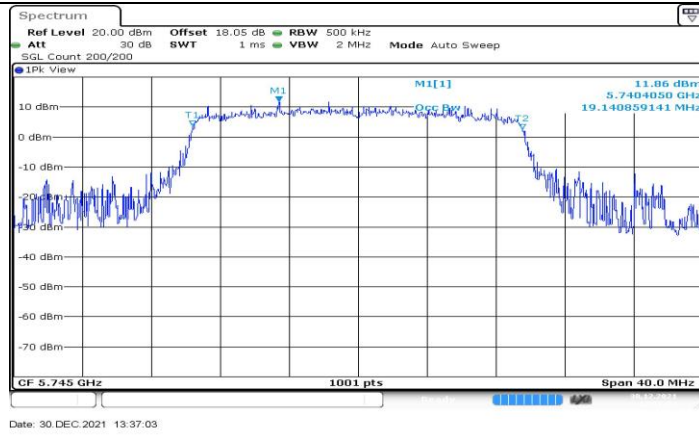
11AX20MIMO Ant2 5745
