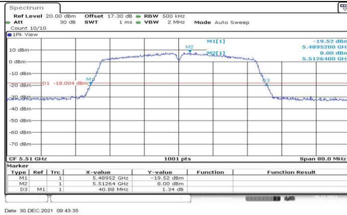
11N40MIMO Ant1 5510
