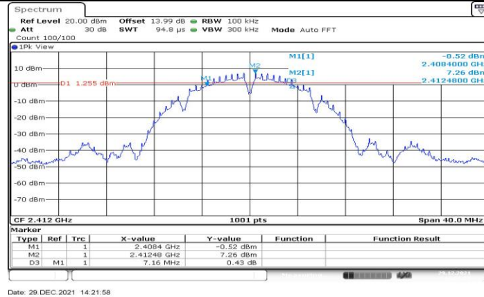
11B_Ant2_2412
