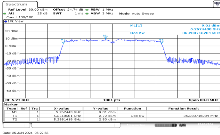
11N40MIMO_Ant1_5270
