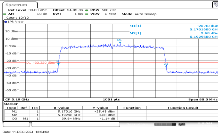
11AX40MIMO_Ant1_5190
