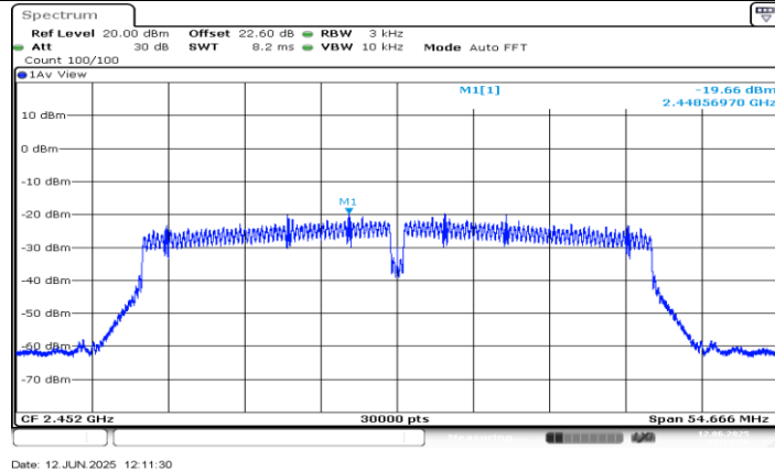
11N40SISO_Ant0_2452
