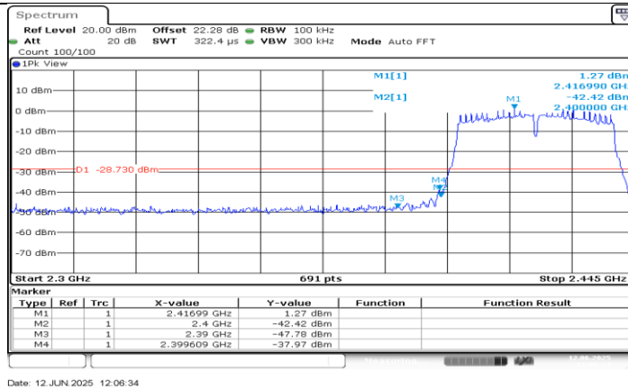
11N40SISO_Ant0_Low_2422
