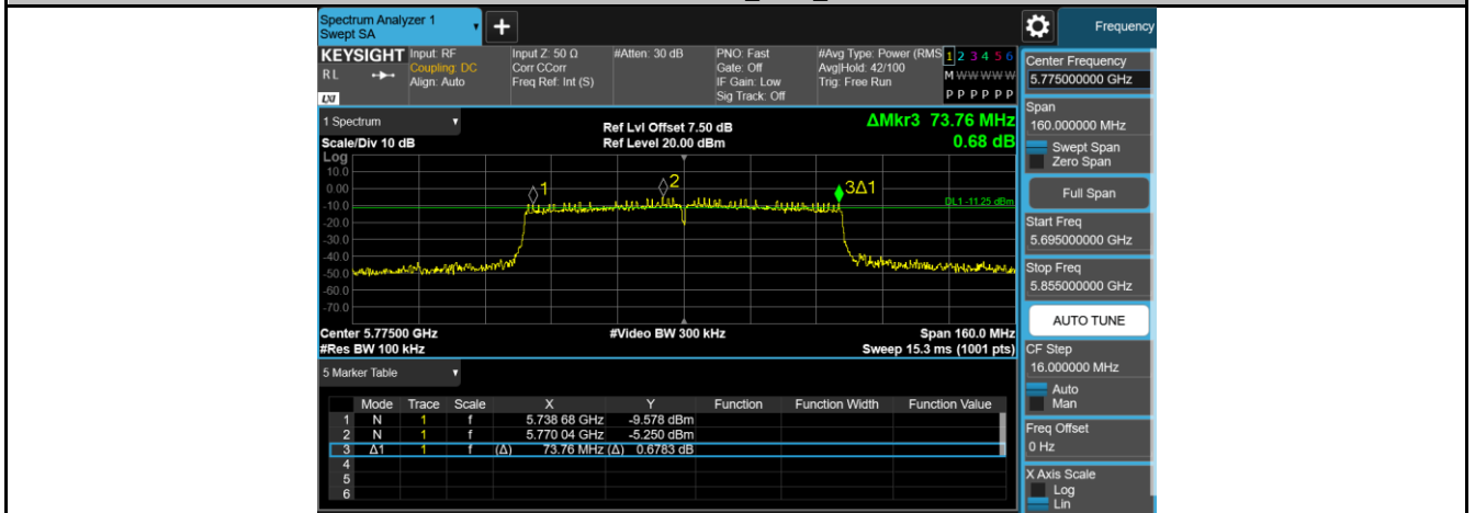
11AC80MIMO_Ant1_5775
