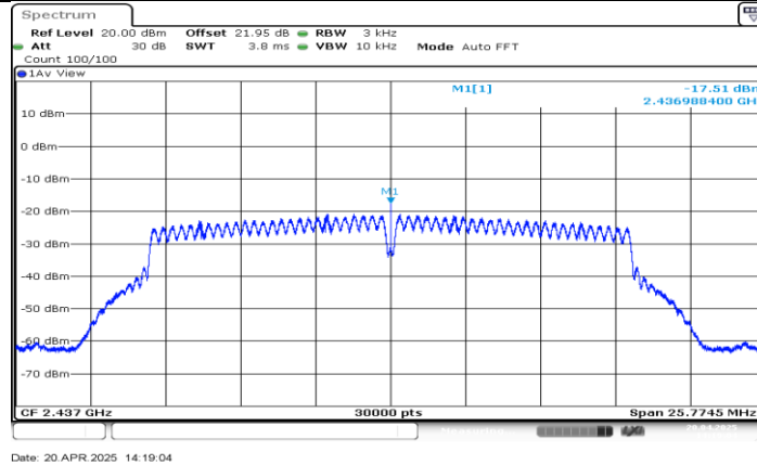
11G_Ant0_2437
