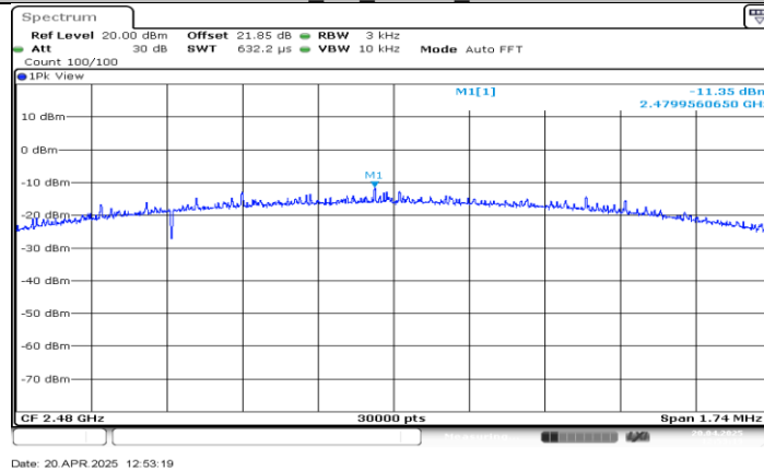
BLE_2M_Ant BT_2480
