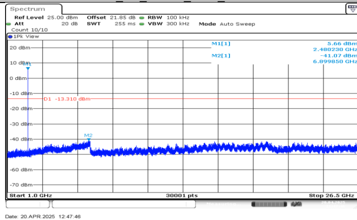
BLE_1M_Ant BT_2480_1000-26500
