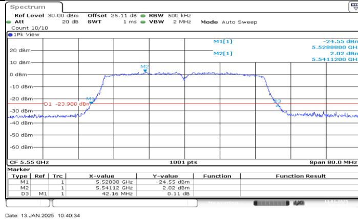
11N40MIMO_Ant0_5550
