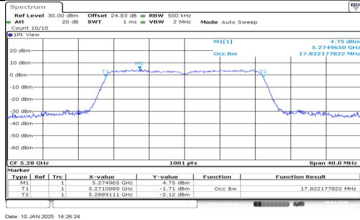
11N20MIMO_Ant1_5280
