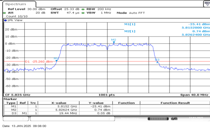
11N20MIMO_Ant0_5825
