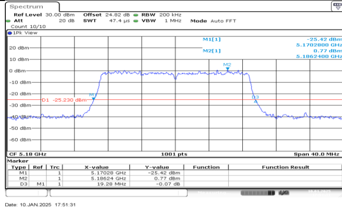
11N20MIMO Ant0 5180
