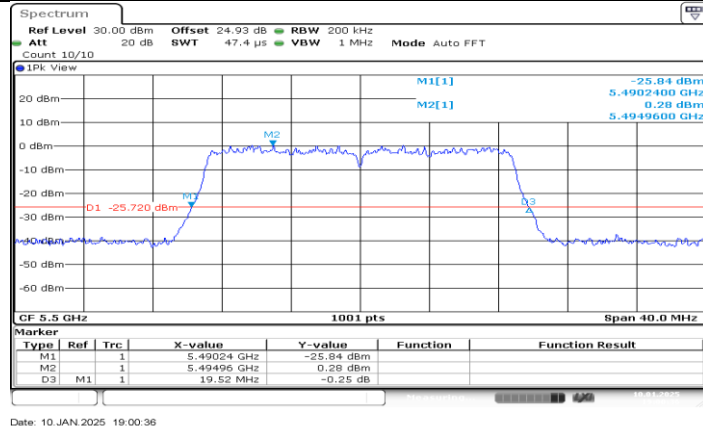
11N20MIMO_Ant0_5500
