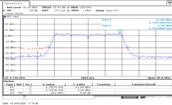
11A_Ant0_5745
