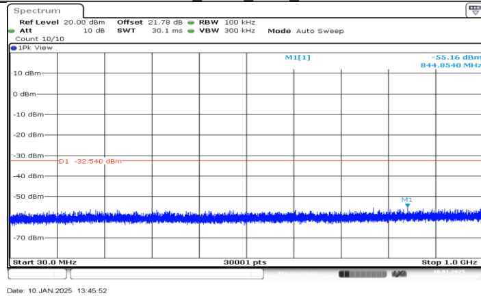
11N40MIMO_ANT0_2422_30-1000
