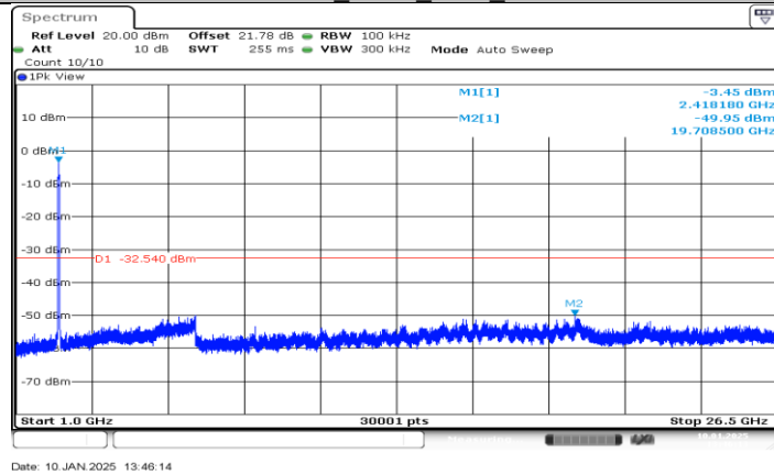
11N40MIMO_ANT0_2422_1000-26500
