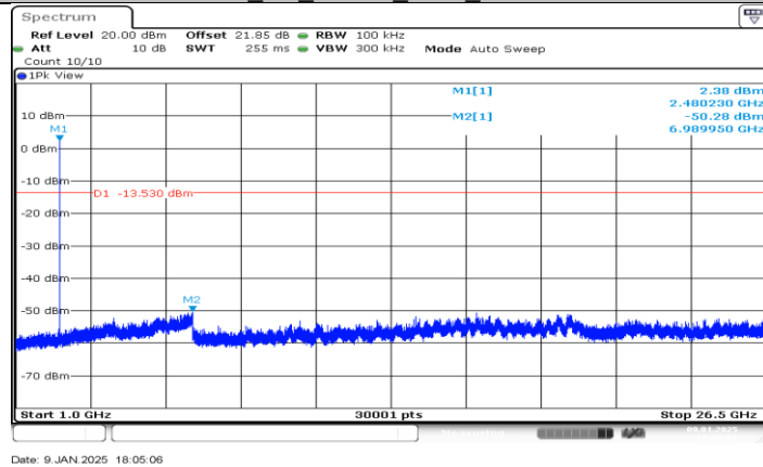
BLE_2M_Ant BT_2480_1000-26500
