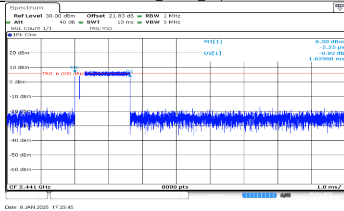
3DH3_Ant BT_Hop
