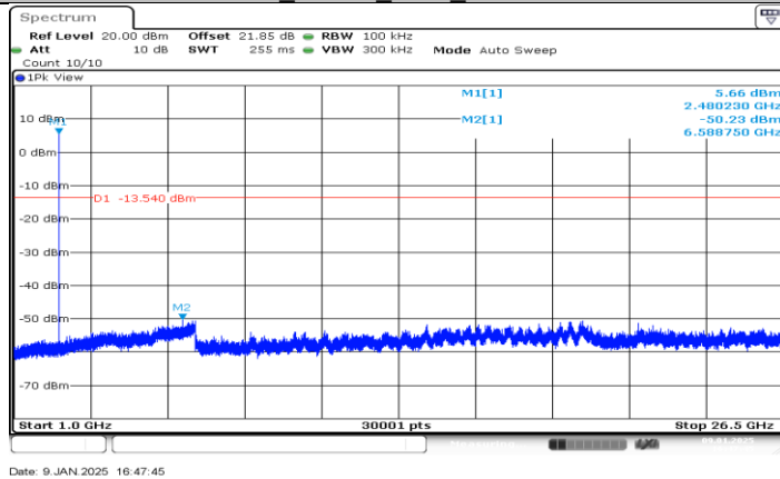
DH5_Ant BT_2480_1000~26500
