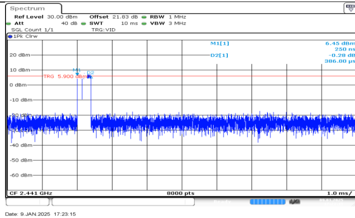
3DH1_Ant BT_Hop
