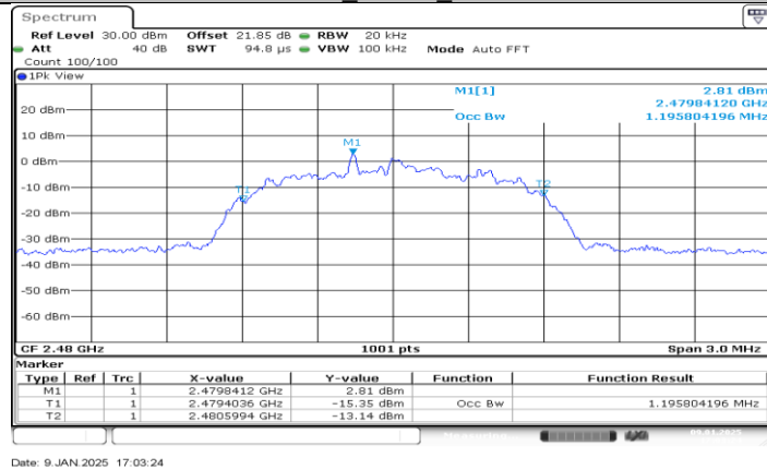
3DH5_Ant BT_2480
