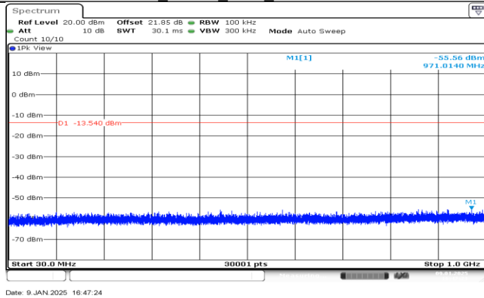
DH5_Ant BT_2480_30~1000
