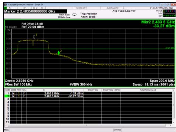
Bandedge-CH09
