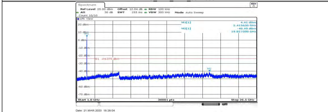
11N20MIMO_Ant1_2412_1000~26500
