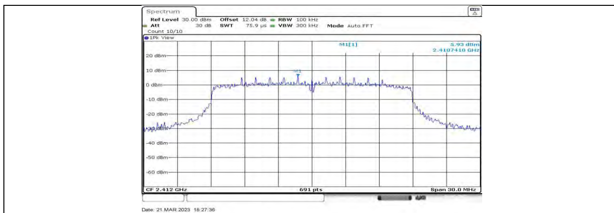
11N20MIMO_Ant1_2412_0~Reference
