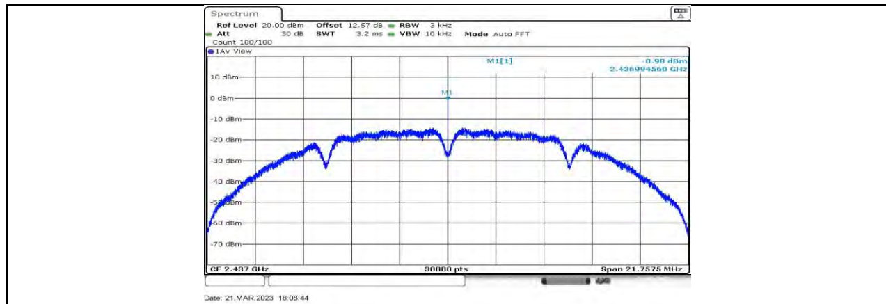
11B_Ant2_2437
