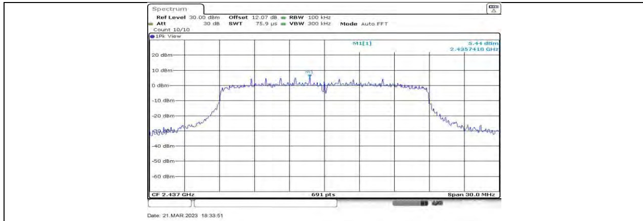
11N20MIMO_Ant1_2437_0~Reference
