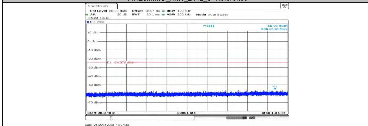
11N20MIMO_Ant1_2412_30~1000
