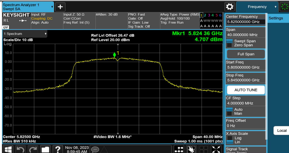
11A_Ant2_5825
