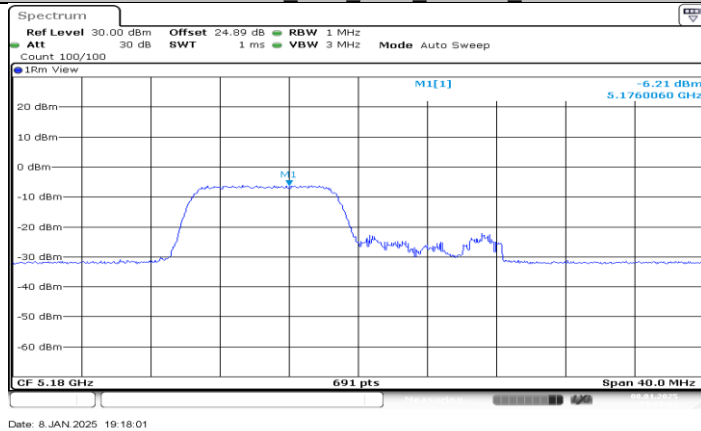
11AX20MIMO_Ant2_5180_106Tone_RU53
