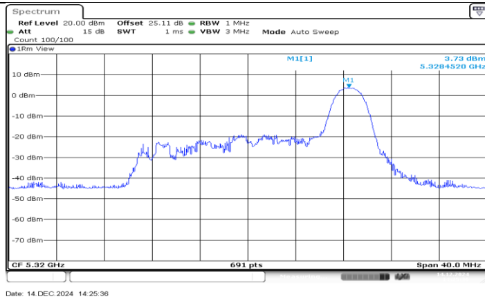
11AX20MIMO_Ant2_5320_26Tone_RU8
