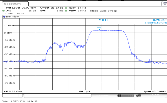
11AX20MIMO_Ant2_5320_106Tone_RU54
