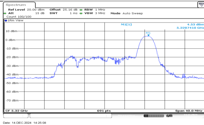
11AX20MIMO_Ant1_5320_26Tone_RU8
