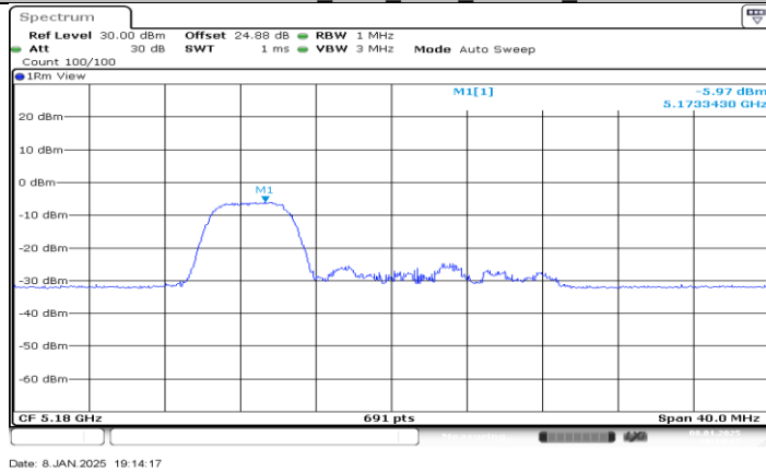
11AX20MIMO_Ant2_5180_52Tone_RU37
