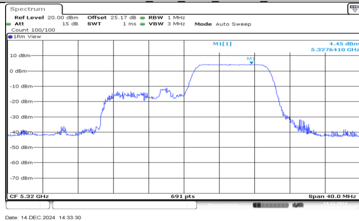
11AX20MIMO_Ant1_5320_106Tone_RU54
