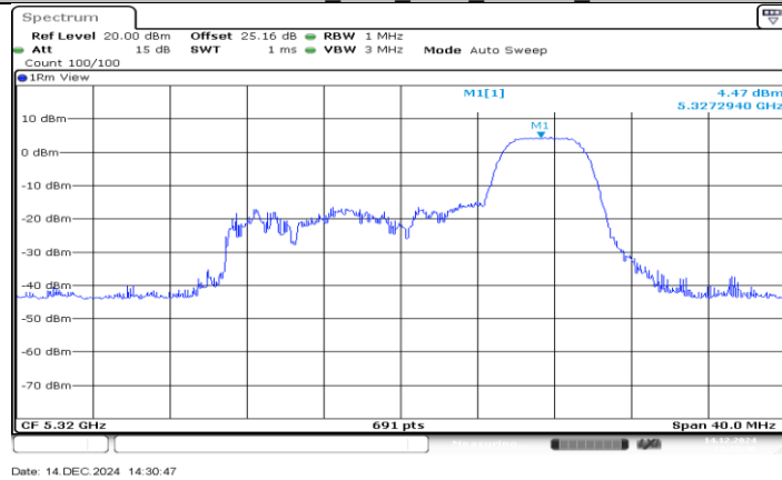
11AX20MIMO_Ant1_5320_52Tone_RU40
