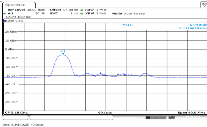
11AX20MIMO_Ant2_5180_26Tone_RU0
