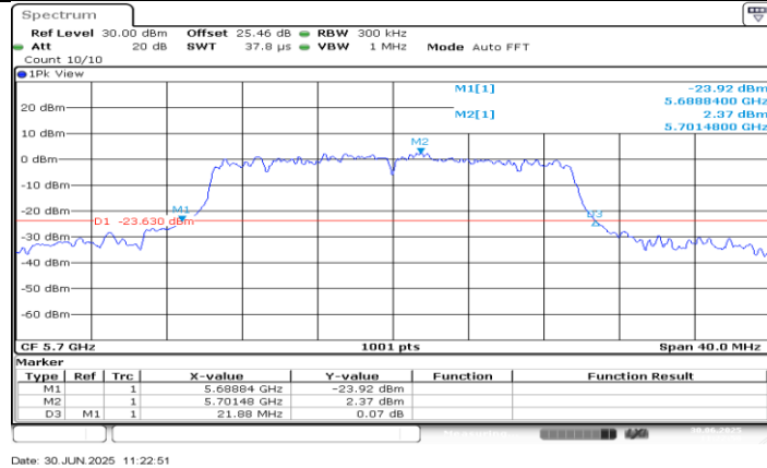
11AX20MIMO_Ant2_5700
