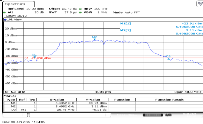
11N20MIMO_Ant1_5500
